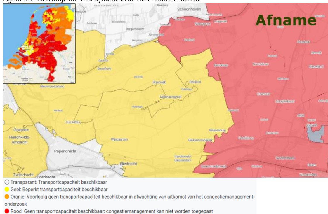
Figuur 6.1: Netcongestie voor afname in de RES Alblasserwaard
